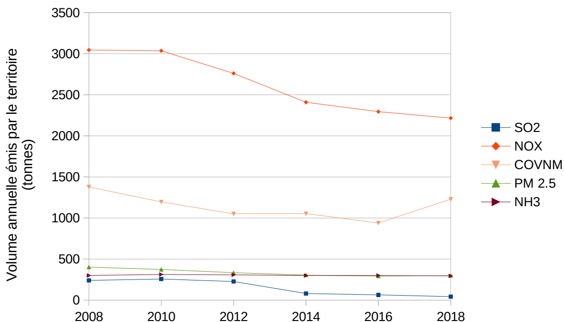
Émissions de polluants par le territoire du CRTE du Sud-Est Saône-et-Loire sur la période 2008-2018
